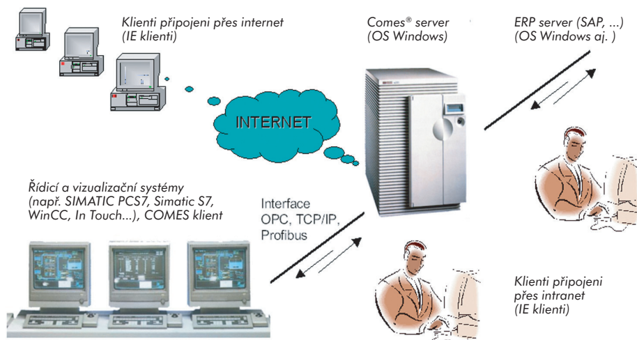
Architektura systému COMES s uživatelským rozhraním Internet Explorer
